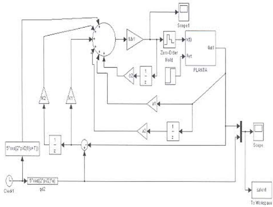
Fig. 2. Diagrama de simulación de estrategia de control discreto particionado. Entrada r(k)=5\cos\pi k T para T=4\text{ms} .
