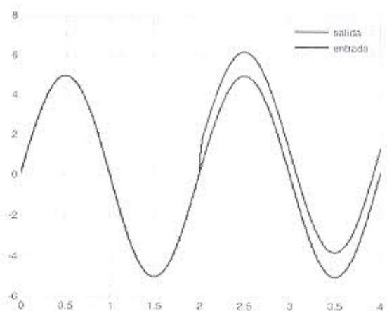
Fig. 5. Entrada y salida de lazo cerrado utilizando controlador discreto particionado. Entrada r(k)=5\text{sen}\pi kT y perturbación constante para T=4\text{msg}
