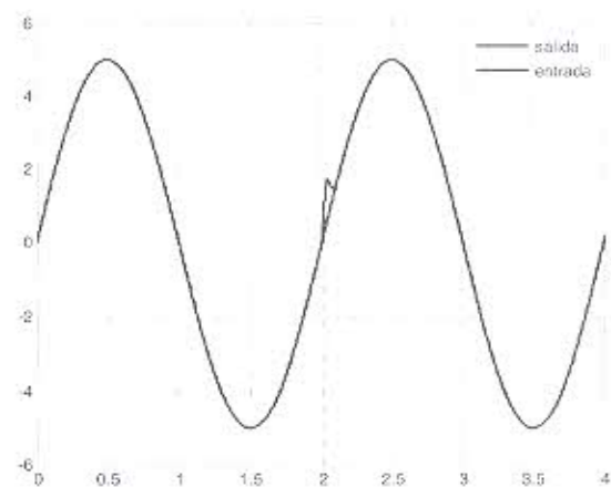
Fig. 9. Entrada y salida de lazo cerrado utilizando controlador discreto particionado con integrador. Entrada r(k)=5\sin\pi kT y perturbación constante para T=4\text{msg}
