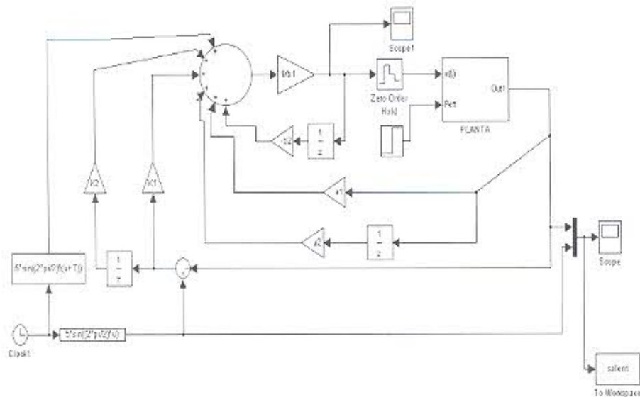
Fig. 1. Diagrama de simulación de estrategia de control discreto particionado. Entrada r(k) = 5 \text{sen} \pi k T para T = 4 \text{ms} .
