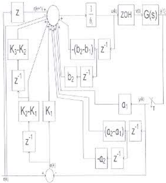
Fig. 2. Estrategia de control discreto con integrador, diagrama de simulación
