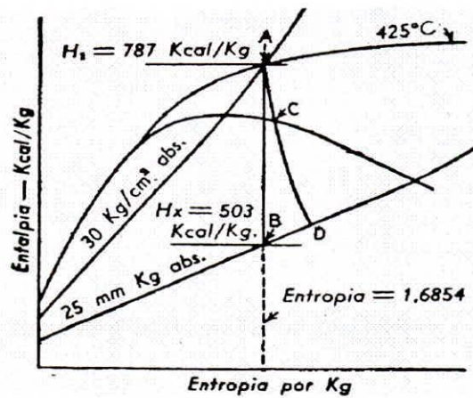
Fig.8. Típica curva de expansión de una turbina
