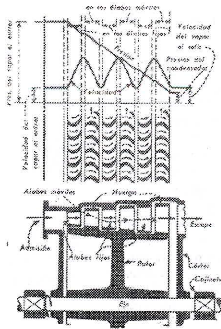
Fig. 03. Turbina de reacción (Parsons).
