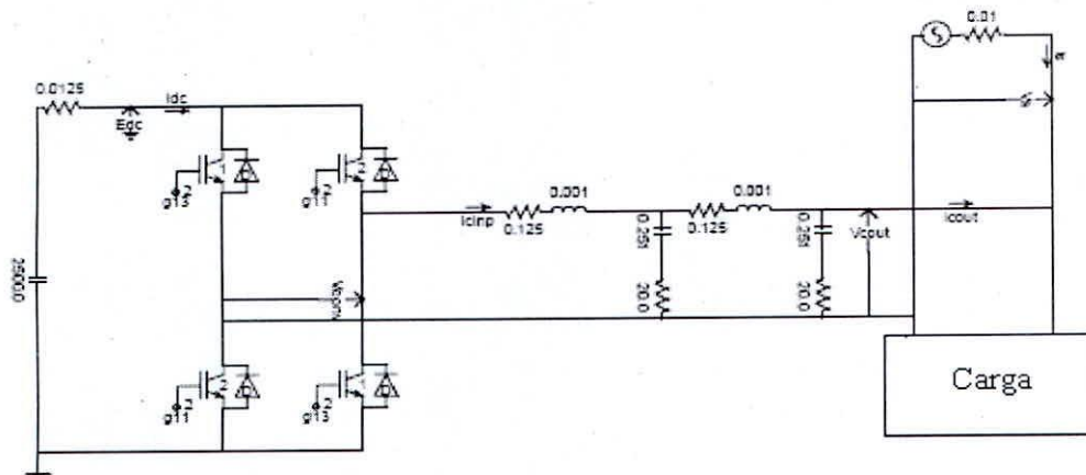
Fig. 4. Filtro Activo de Potencia, carga y red de alimentación
