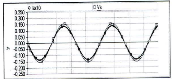
Fig.17 Tensión Vs y Corriente Is de línea con Filtro Activo de Potencia.
