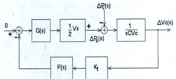
Fig.3 Modelo para el análisis de Potencia Real
