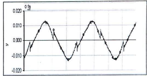
Fig. 11. Formas de onda de la señal de modulación generada por el control.
