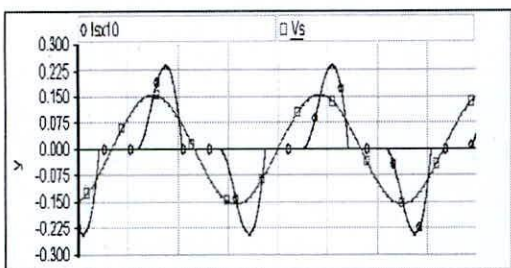
Fig. 6. Tensión Vs y Corriente Is de línea del rectificador.
