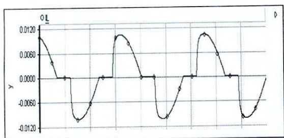
Fig. 27. Formas de onda de la corriente i_L en los terminales de entrada del rectificador monofásico
