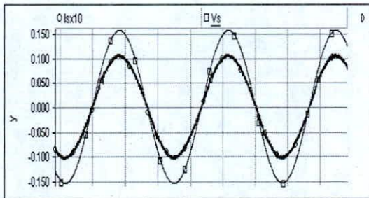
Fig. 33. Tensión V_s y Corriente I_s de línea con Filtro Activo de Potencia
