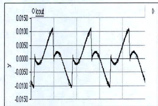
Fig. 36. Formas de onda de la corriente de salida del FAP e inyectada en los terminales de entrada del rectificador
