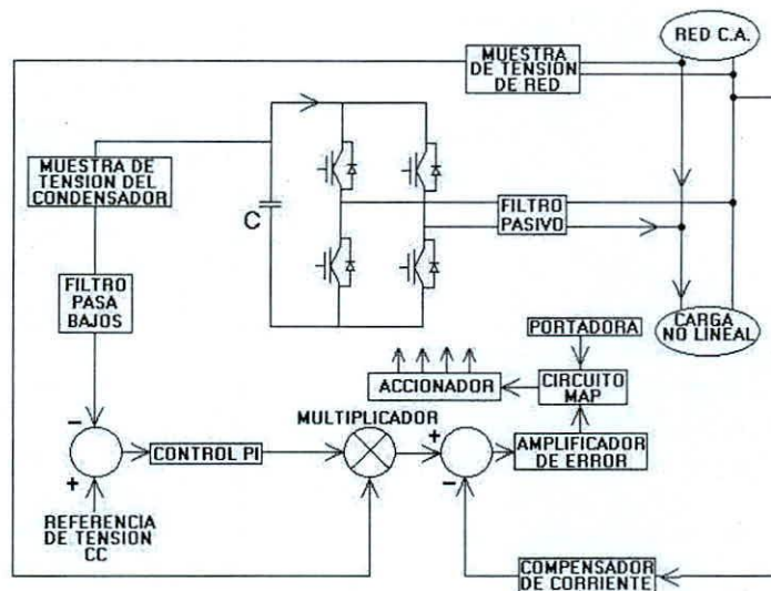
Fig. 1. Diagrama de Bloques del Filtro Activo de Potencia Monofásico Paralelo
