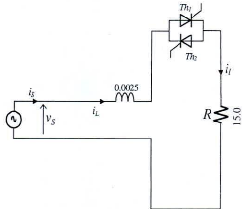
Fig. 24. Convertidor AC-AC monofásico sin FAP.
