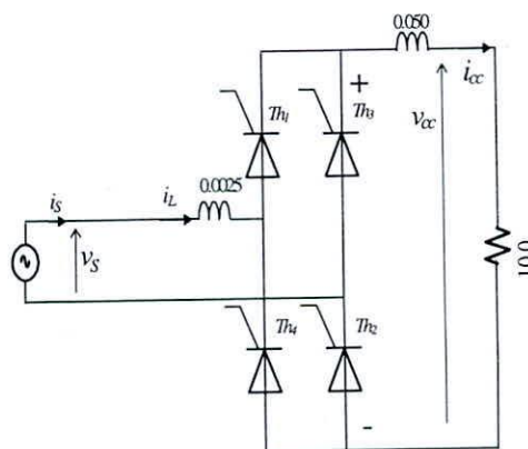
Fig. 31. Rectificador monofásico controlado sin FAP.
