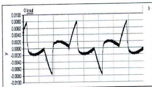
Fig. 29. Formas de onda de la corriente de salida del FAP e inyectada en los terminales de entrada del rectificador
