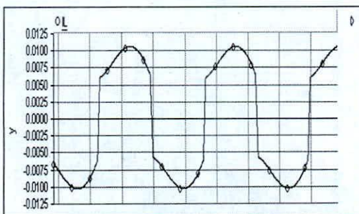
Fig. 34. Formas de onda de la corriente I_L en los terminales de entrada del rectificador monofásico.
