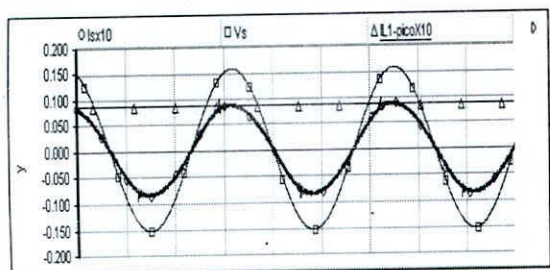
Fig. 26. Tensión V_s y Corriente I_s de línea con Filtro Activo de Potencia
