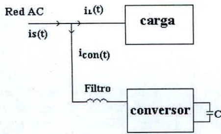
Fig. 2. Circuito de Potencia del FAP
