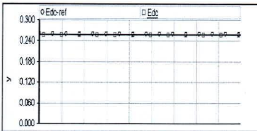
Fig. 21. Tensión de referencia y Tensión en el DC link del inversor en 260 V.
