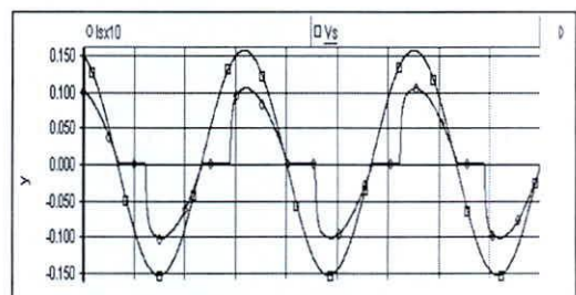
Fig. 25. Tensión Vs y Corriente Is de línea sin filtro Activo de Potencia
