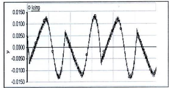
Fig. 12. Formas de onda de la corriente de entrada al filtro pasivo
