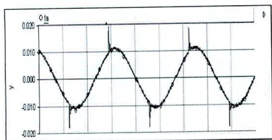
Fig. 28. Formas de onda de la señal de modulación generada por el control.
