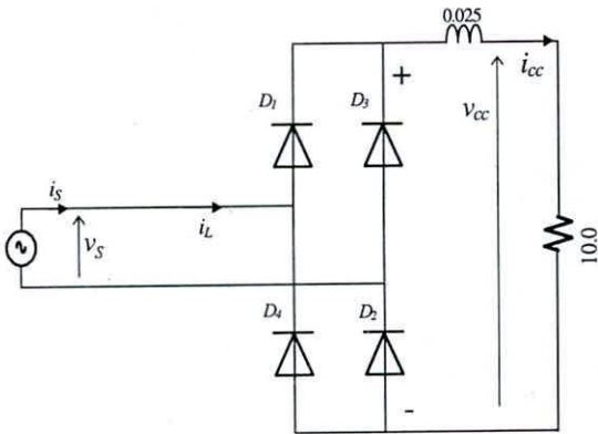
Fig. 15. Rectificador monofásico con filtro inductivo y sin FAP
