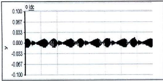
Fig. 8. Formas de onda de la corriente en el condensador en los terminales DC del inversor, donde se verifica que tiene valor medio cero.
