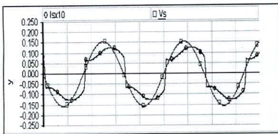
Fig. 16. Tensión Vs y Corriente Is de línea sin filtro Activo de Potencia
