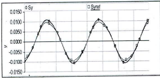
Fig. 14. Formas de onda de las señales de referencia de corriente y corriente real entregada por la red.
