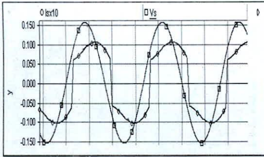
Fig. 32. Tensión V_s y Corriente I_s de línea sin Filtro Activo de Potencia.
