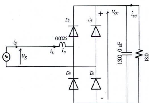
Fig. 5. Rectificador monofásico con filtro por condensador y sin FAP.
