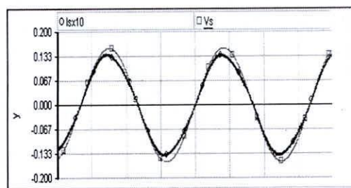
Fig. 7. Formas de onda de tensión Vs y Corriente Is de línea luego de la compensación efectuada por el filtro activo.
