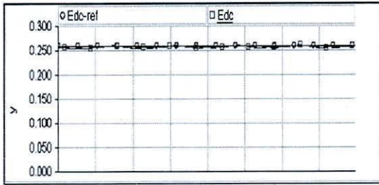
Fig. 9. Tensión de referencia y Tensión en el DC link del Inversor en 260 V.
