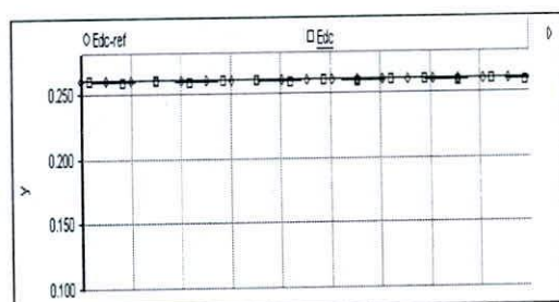
Fig. 30. Tensión de referencia y Tensión en el DC link del inversor en 260 V.
