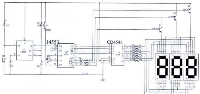
Figura 4. Módulo de contador independiente
