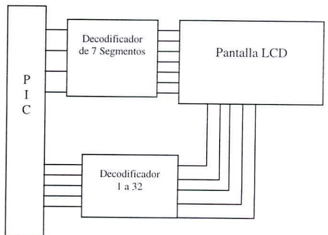
Figura 6. Diagrama de bloques del Contador Hematológico utilizando microcontrolador PIC.
