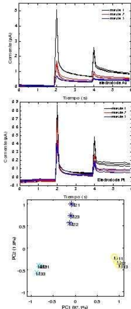
Fig. 7. a) La respuesta de corriente en función del tiempo para las muestras de agua contaminada para los electrodos de Au y Pt, and b) la gráfica de componentes principales para el electrodo de Au.
