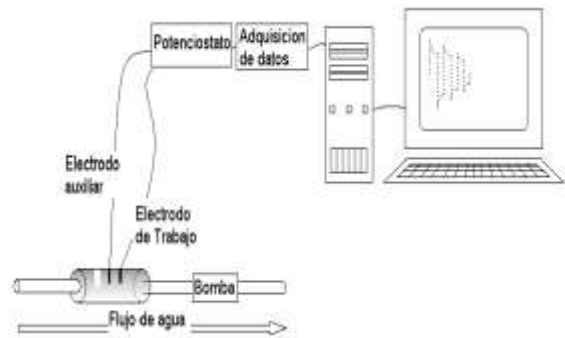
Fig. 2. Diagrama esquemático del sistema de calidad de agua desarrollada.
