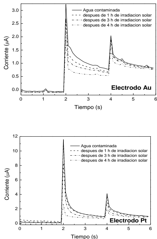
Fig. 8. La respuesta de corriente en función del tiempo para las muestras de agua contaminada para los electrodos de Au y Pt, sometidas diferentes tiempos de irradiación solar.
