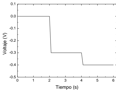
Fig. 6. El voltaje en función del tiempo utilizado para el análisis de agua.
