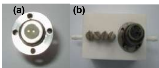
Fig. 3. Fotografías a) de la parte superior del cabezal sensor y b) de la cámara de medida.
