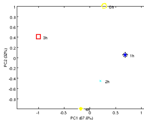
Fig. 9. Gráfica de componentes principales para el electrodo de Au de muestras de agua del río Yaurisque con diferentes tiempos de irradiación solar.
