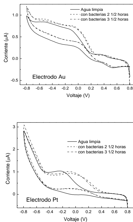
Fig. 5. Voltametría cíclica del agua limpia y contaminada con E. coli para el electrodo de oro (a) y platino (b).
