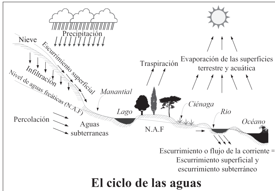
Figura 1. Ciclo hidrológico.
