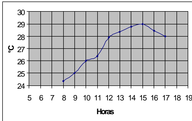
Figura 4. Evolución de la temperatura del agua en la piscina
