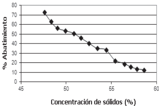
Figura N.º 15. Abatimiento en función de la concentración de sólidos de pasta mineral de relave de manganeso.
