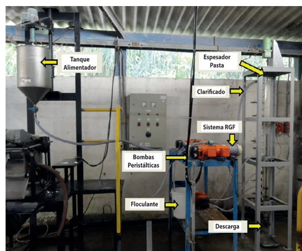
Figura N.º 2. Vista general del montaje de operación del espesador de pasta desarrollado. (Barreda, 2012).
