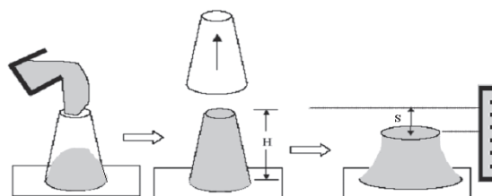
Figura N.º 4. Procedimiento del ensayo de abatimiento ("slump"). (Clayton et al, 2003).
