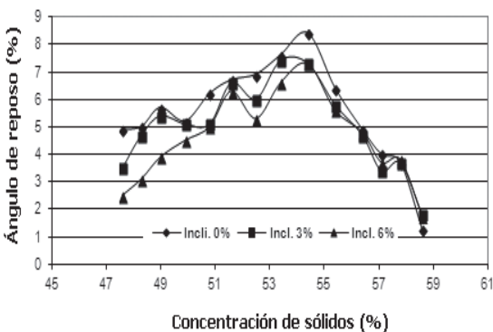
Figura N.º 16. Ángulo de reposo versus concentración de sólidos de las pastas minerales de relaves de manganeso.
