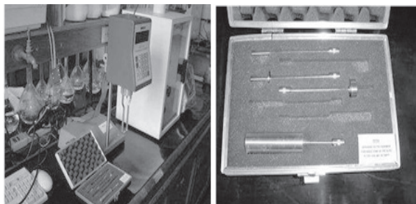
Figura N.º 6. Viscosímetro Brookfield modelo DV-III con sus “spindles” LV-1, LV-2, LV-3 y LV-4.
