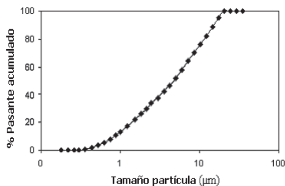
Figura N.º 7. Distribución granulométrica de la muestra mineral.
