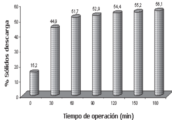
Figura N.º 14. Variación de % de sólidos de la descarga en función del tiempo de operación para las mejores condiciones operacionales continuas.
