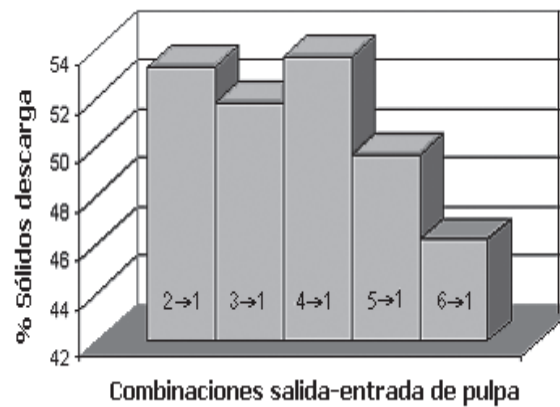
Figura N.º 13. Variación de los porcentajes de sólidos en peso en función de las combinaciones de los agujeros con el tiempo de residencia de 10min, adición de 50gpt de floculante y volumen de pulpa de 7L.
