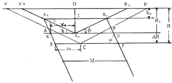
Figura N° 5. Determinación de la dirección de profundización óptima de tajo a cielo abierto a la profundidad H < H2.
