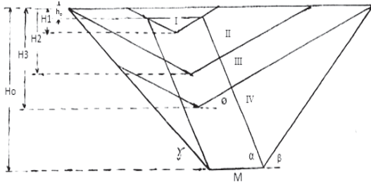
Figura N.º 2. Yacimiento mineral tabular equivalente con sus variables y dividido en Etapas de profundización: I, II, III, IV
