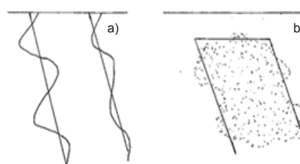
Figura N.º 1. Formas equivalentes de contornos de yacimientos irregulares inclinados convertidos en regulares: a) Cuerpo tabular masivo, b) Yacimiento diseminado
