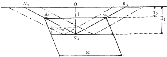
Figura 4. Dirección óptima de profundización de un tajo a C.A. en un yacimiento tabular equivalente. Fase I.
