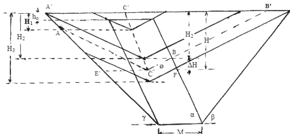
Figura N.º 6. Determinación de la dirección de profundización óptima de tajo a cielo abierto en el intervalo H_2 < H < H_3 .
