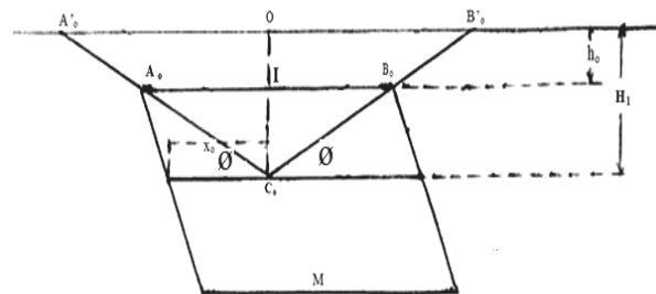
Figura N.º 3. Primera Fase. Determinación de profundidad H_1 y parámetro X_0 que ubican el vértice C_0 de la excavación de máxima extracción.
