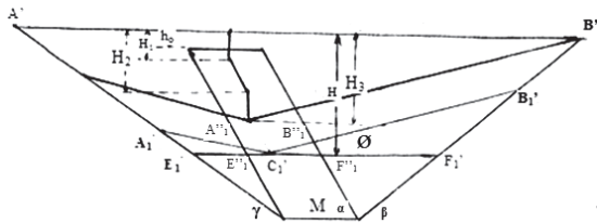
Figura N.º 7. Determinación de la dirección de profundización de tajo a cielo abierto en la IV zona H \leq H_4 .
