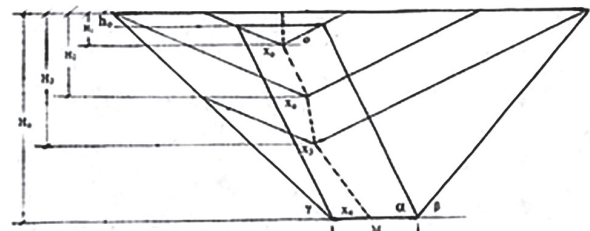
Figura N.º 8. Dirección óptima de profundización del tajo a cielo abierto para los datos del yacimiento dado.
