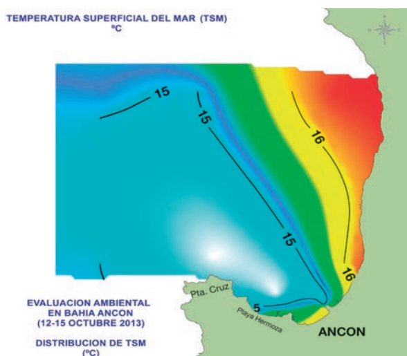
Figura N° 4. Distribución de la temperatura superficial del mar. Fuente: Elaboración propia.
