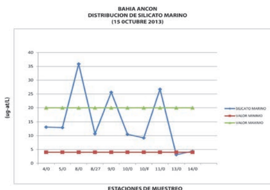
Figura N° 17. Distribución del silicato y valores ECA en agua de mar bahía Ancón. Fuente: Elaboración propia
