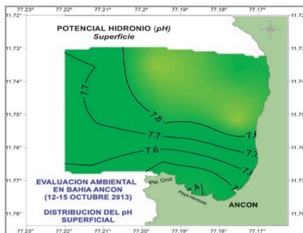
Figura N° 13. Distribución superficial de valores de pH en bahía Ancón 12-15 octubre 2013. Fuente: Elaboración propia
