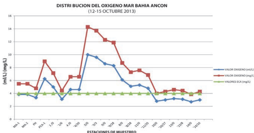
Figura N° 7. Distribución del oxígeno superficial y fondo comparada con el ECA D.S. 002-2008 –MINAM. Fuente: Elaboración propia
