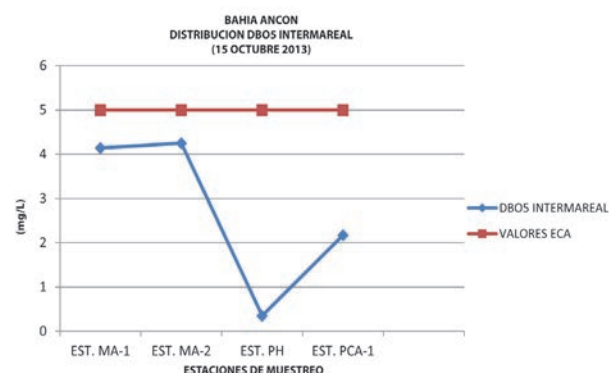
Figura Nº 10. Demanda Bioquímica de Oxígeno (DBO5) en zona intermareal B. Ancón. Fuente: Elaboración propia
