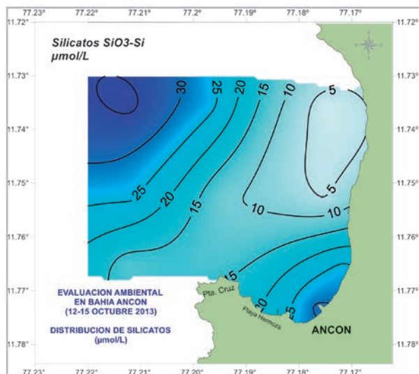
Figura N° 18. Distribución del silicato superficial en agua de mar bahía Ancón. Fuente: Elaboración propia
