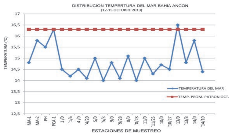
Figura N° 6. Temperatura superficial del mar. Fuente: Elaboración propia
