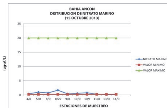
Figura 19. Distribución de los nitratos en bahía Ancón. Fuente: Elaboración propia
