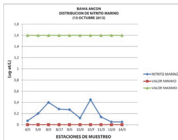
Figura 20. Distribución de los nitritos en bahía Ancón. Fuente: Elaboración propia
