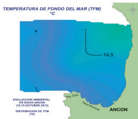
Fig. N° 5. Distribución de la temperatura del fondo del mar. Fuente: Elaboración propia
