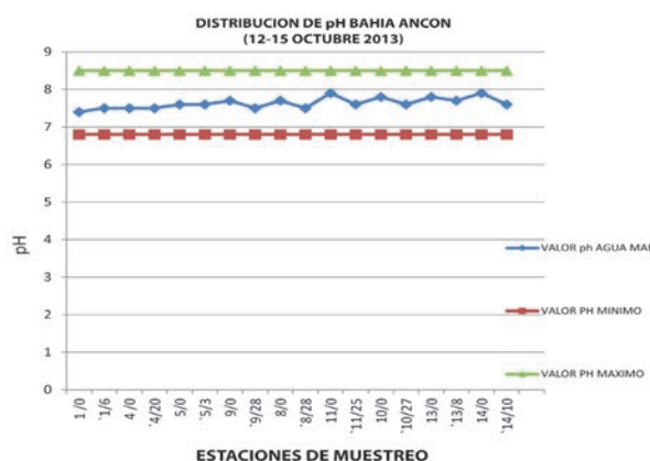
Figura N° 14. Distribución superficial de valores de pH con ECA de pH en Bahía Ancón 12-15 octubre 2013. Fuente: Elaboración propia
