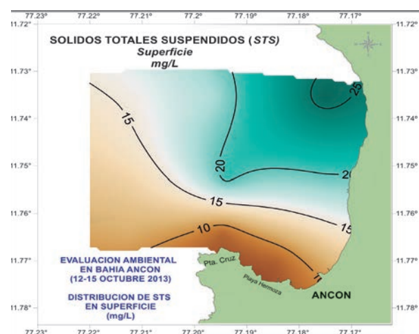
Figura Nº 11. Distribución del STS superficial del mar en bahía Ancón. Fuente: Elaboración propia
