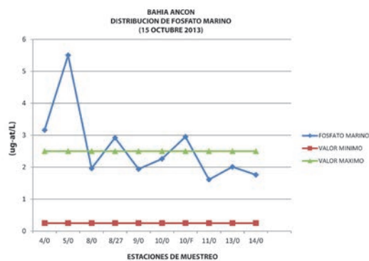
Figura N° 15. Distribución del fosfato y valores ECA en Bahía Ancón.
