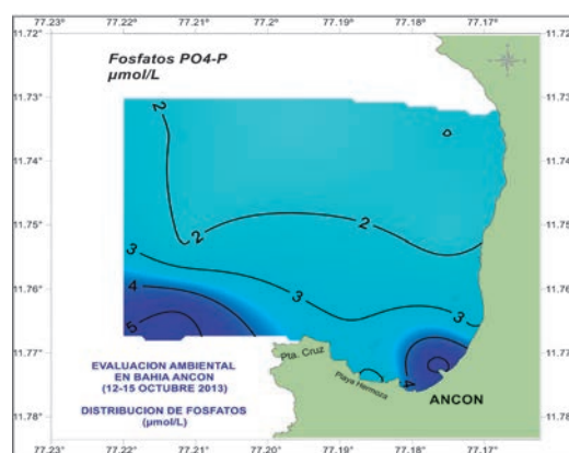
Figura N° 16. Distribución del fosfato superficial en Bahía Ancón 12-15 octubre 2013.
