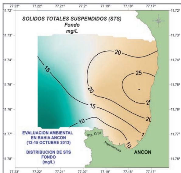
Figura N° 12. Distribución del STS de fondo del mar en bahía Ancón 12-15 octubre de 2013. Fuente: Elaboración propia
