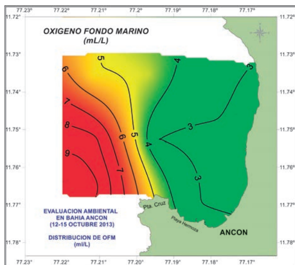
Figura Nº 8. Distribución del oxígeno superficial del mar en bahía Ancón 12-15 octubre de 2013. Fuente: Elaboración propia
