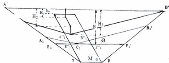
Figura N° 7. Determinación de la dirección de profundización de tajo a cielo abierto en la IV zona H ≤ H4.
