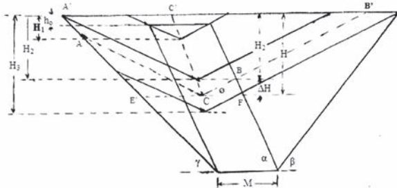
Figura N° 6. Determinación de la dirección de profundización óptima de tajo a cielo abierto en el intervalo H2 < H ≤ H3.
