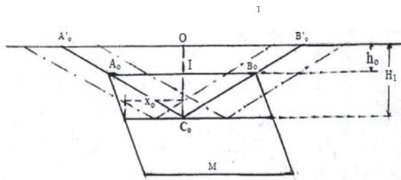
Figura N° 4. Dirección óptima de profundización de un tajo a C. A. en un yacimiento tabular equivalente. Fase I.
