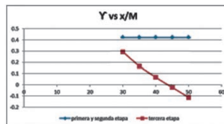
Figura N° 11. \gamma vs. x/M fases 1, 2 y 3.
