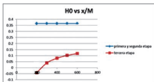
Figura Nº 14. H_0 vs x/M fases 1,2 y 3
