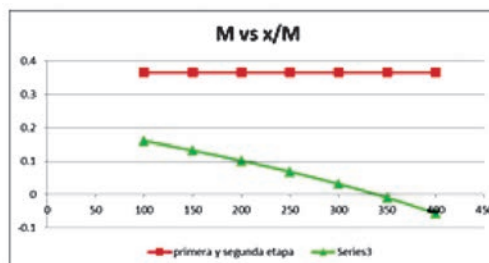
Figura N° 13. M vs. x/M fases 1,2 y 3.
