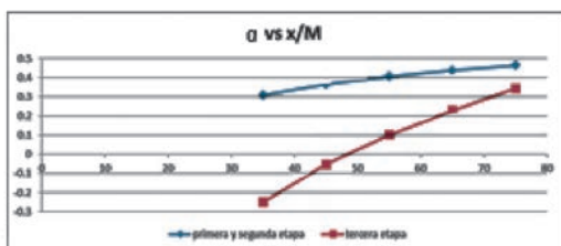
Figura N° 9. \alpha vs x/M de las fases 1,2 y 3.
