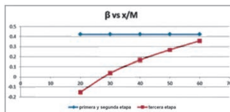
Figura N° 12. \beta vs. x/M fases 1,2 y 3.
