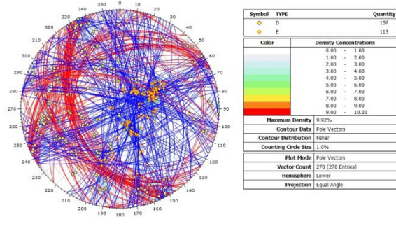
Figura N° 5: Tendencia de las Estructuras en la Formación Pariatambo-270 planos.
