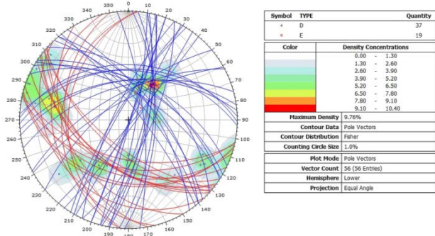
Figura N° 3: Tendencia de las Estructuras en las Formaciones Farrat-Inca-56 planos.
