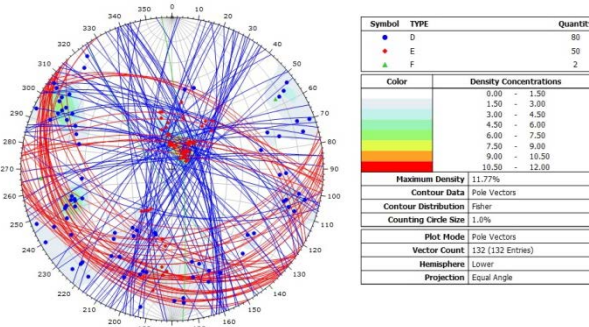
Figura N° 4: Tendencia de las Estructuras en la Formación Chulec-132 planos.
