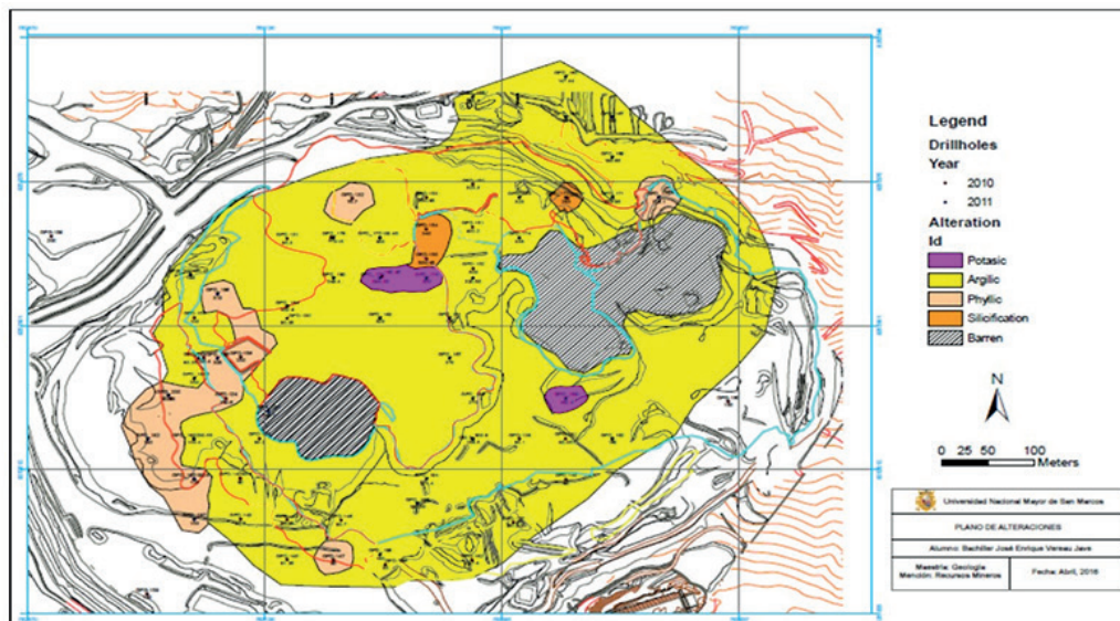
Figura N°5. Mapa de alteraciones hidrotermales. Fuente: Elaboración propia.
