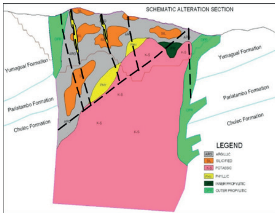
Figura N°7. Esquematación del zoneamiento lateral de las alteraciones en el yacimiento Corona. Geología del Pórfido de Cu – Au, de Cerro Corona, Gold Fields La Cima S.A
