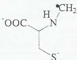
radical dianión
