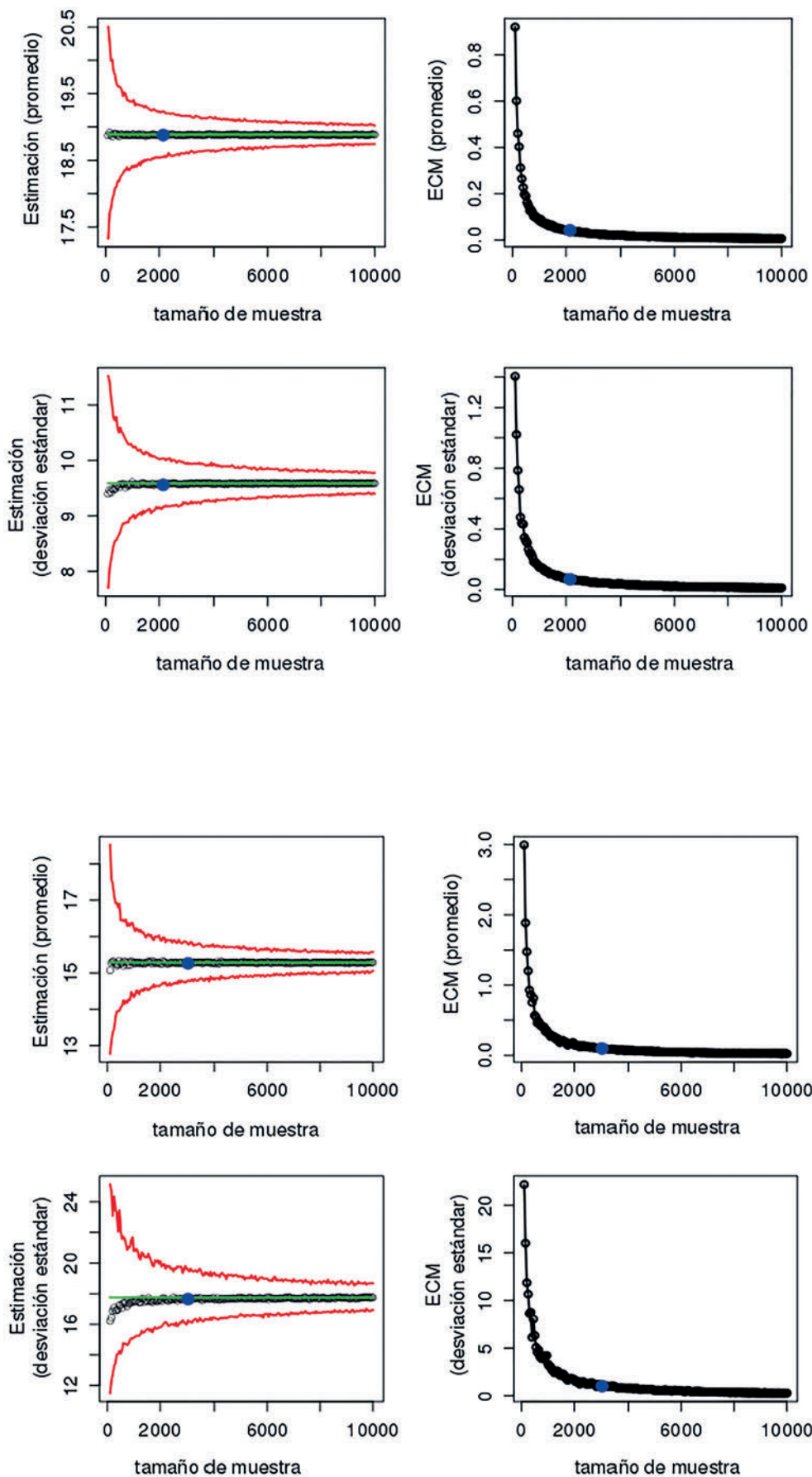
Figura 2.6b. Cálculos de bandas de confianza y error cuadrático medio (ECM) para el promedio y la desviación estándar de la duración del viaje a escala anual, para un ejemplo donde N=57000 . A la izquierda: estimaciones del promedio (arriba) y la desviación estándar (abajo) para cada tamaño de muestra. El valor verdadero está representado por una línea horizontal verde. Las bandas de confianza están en rojo. Los valores estimados se representan por circunferencias negras. A la derecha: error cuadrático medio para el promedio (arriba) y la desviación estándar (abajo), para cada tamaño de muestra. En todos los casos, el valor azul indica el valor óptimo para esa réplica.
