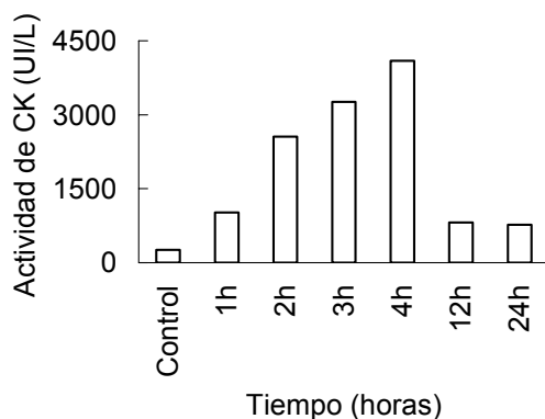
Figura 3. La liberación de creatina quinasa, en el plasma de ratones, se incrementó por efecto de la miotoxina desde la primera hora, alcanzando un valor de 4090 luego de 4 h y disminuyendo a valores casi normales después de 24 h.
