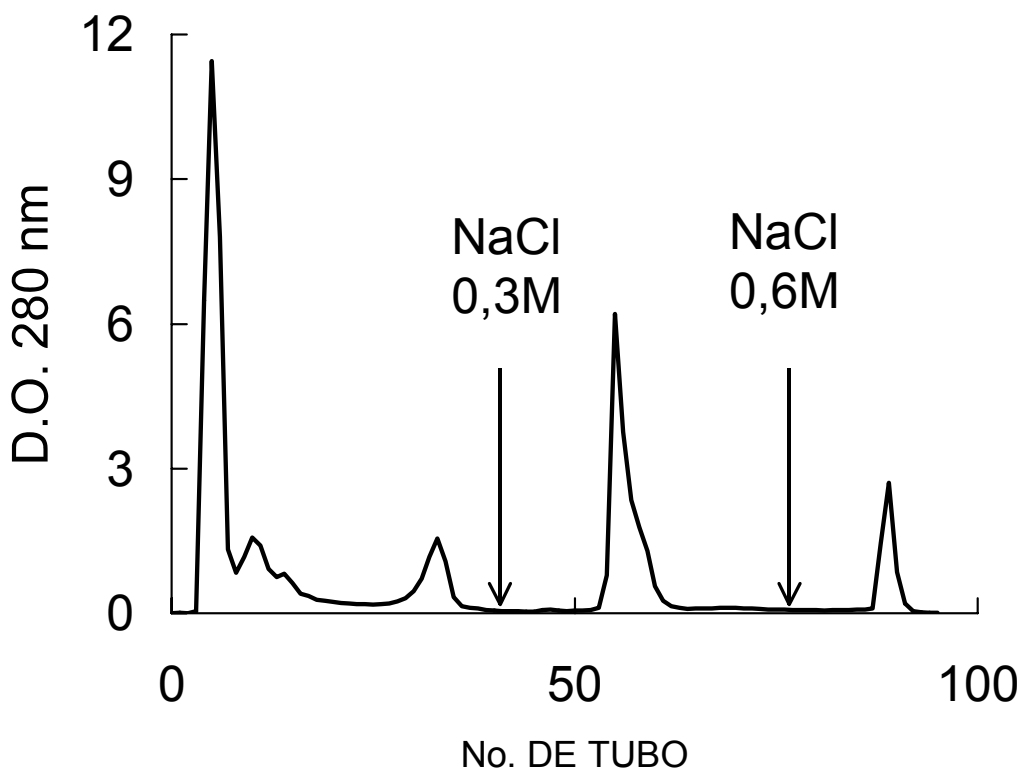
Figura 1. Purificación de la miotoxina. Al pasar el veneno de B. atrox por la columna de CM Sephadex C-50 a pH 7, la miotoxina quedó retenida y fue eluida sólo luego de añadir NaCl 0,6 M al eluyente.
