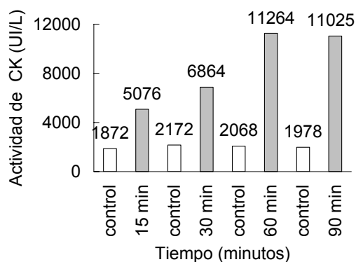
Figura 4. La actividad de la creatina quinasa en músculo aislado con miotoxina, fue dependiente del tiempo de incubación, obteniéndose el valor más alto luego de 1 h.
