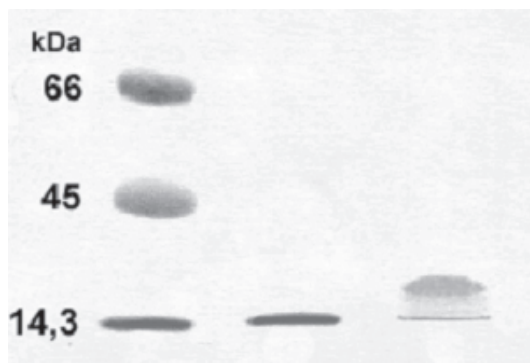
Figura 2. Electroforesis en gel de policrilamida. La PAGE-SDS de la miotoxina aislada mostró la presencia de una banda proteica tanto en condiciones reductoras como no reductoras, pero con diferentes movilidades electroforéticas. En el carril (1) se ven las proteínas albúmina (66 kDa), ovoalbúmina (45 kDa) y lisozima (14,3 kDa); el carril (2) corresponde a la miotoxina reducida (14 kDa) y en el carril (3) se muestra la miotoxina no reducida (25 kDa).
